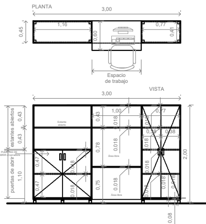
M1 - MUEBLE MDF BOX DE GUARDADO
