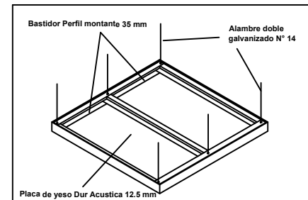
DETALLE MÓDULOS CIELORRASO SUSPENDIDO
