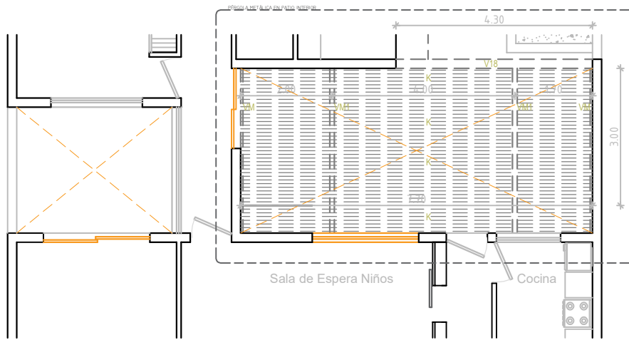
Planta sector
