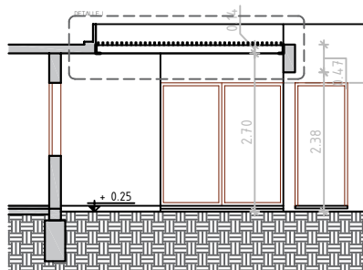
Detalle Patio
