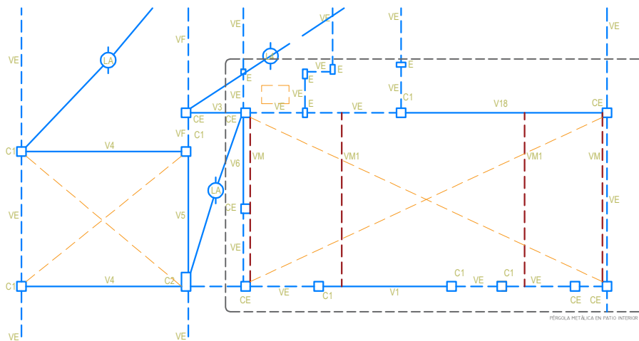
Cubierta Techos
