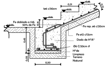
DETALLE ESCALINATA H17 - ADN420
