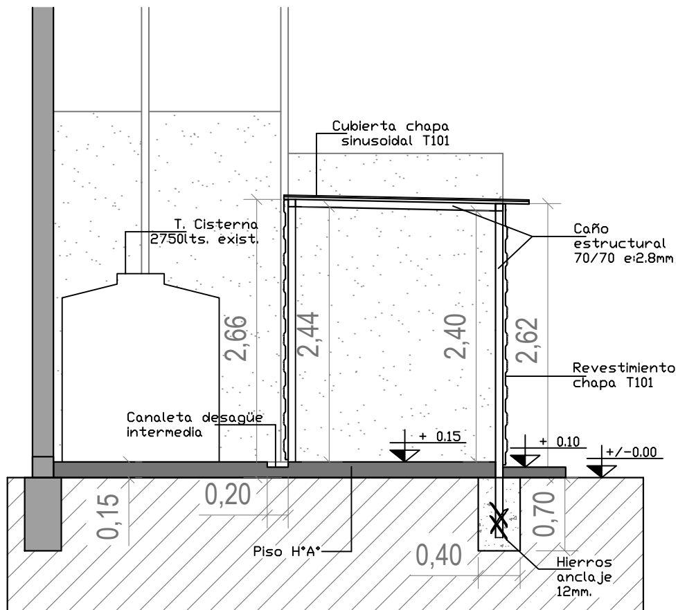
Corte transversal - Esc.:1:50
