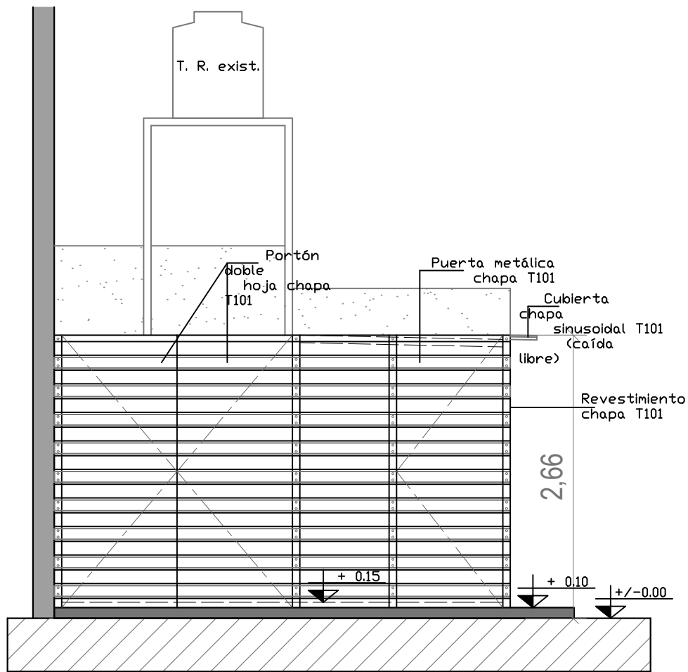
Vista frontal - Esc.:1:50
