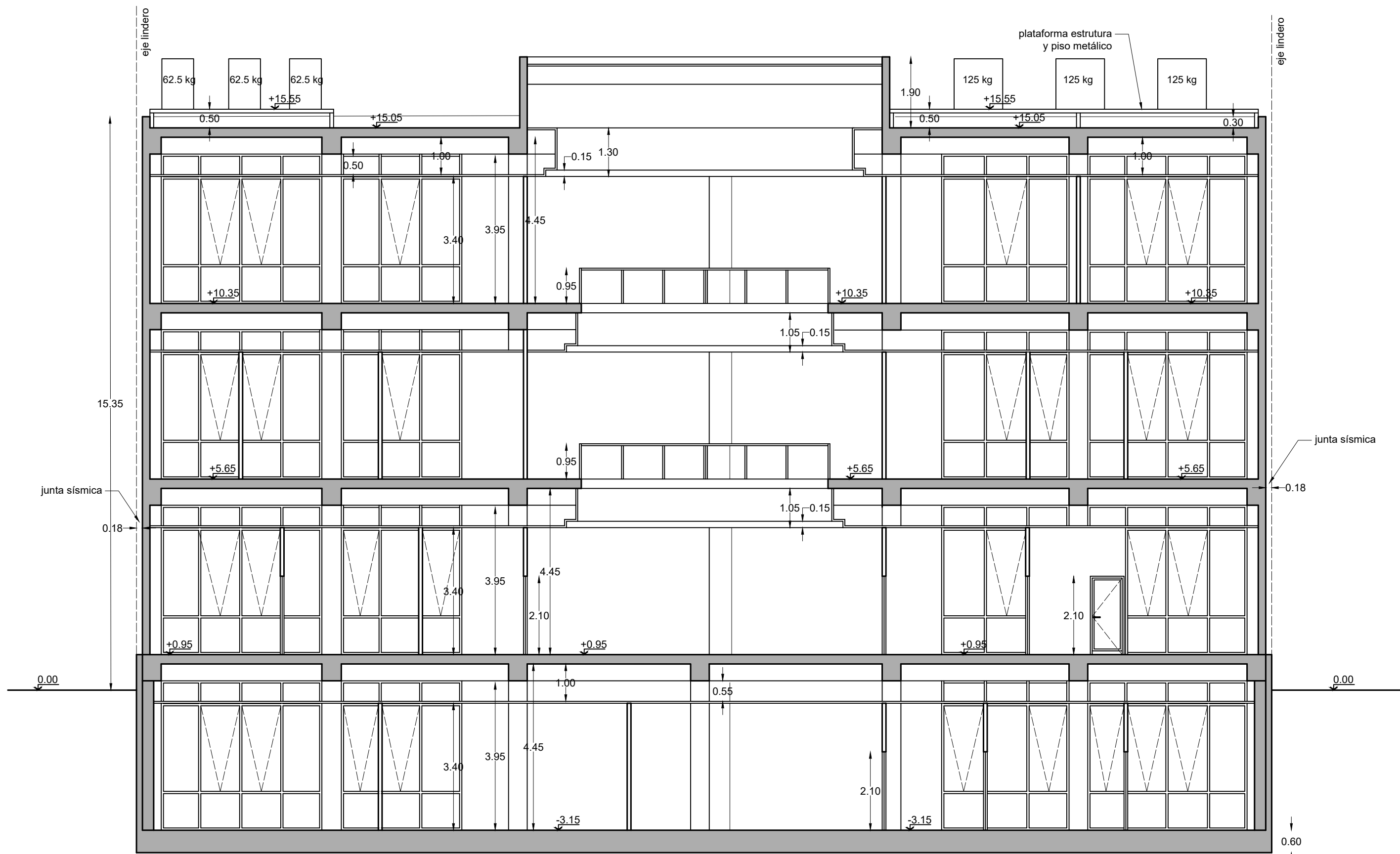
CORTE B-B
