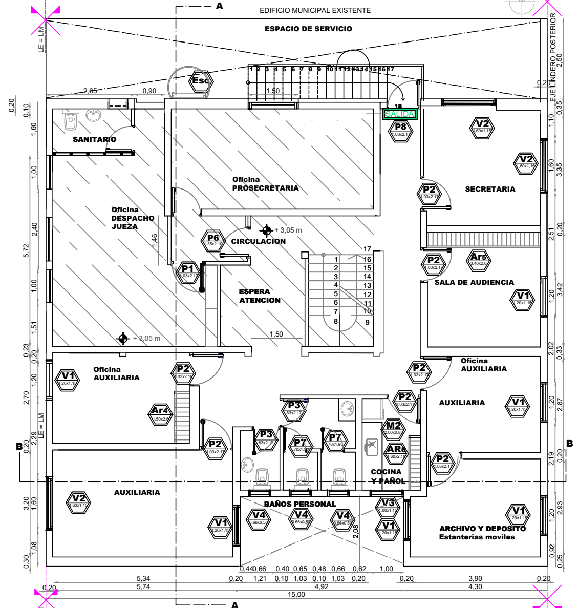
PLANTA ALTA
