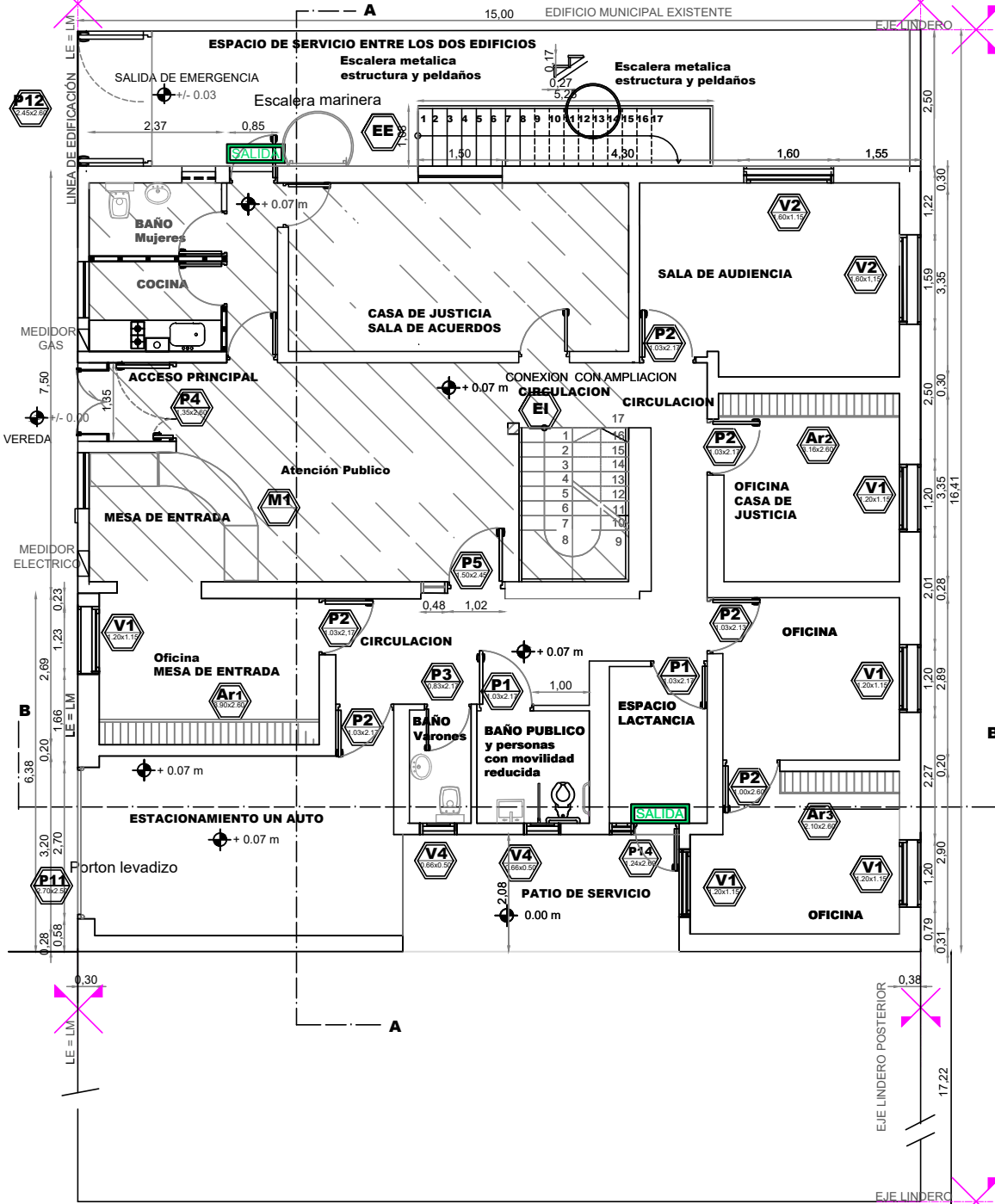
PLANTA BAJA
