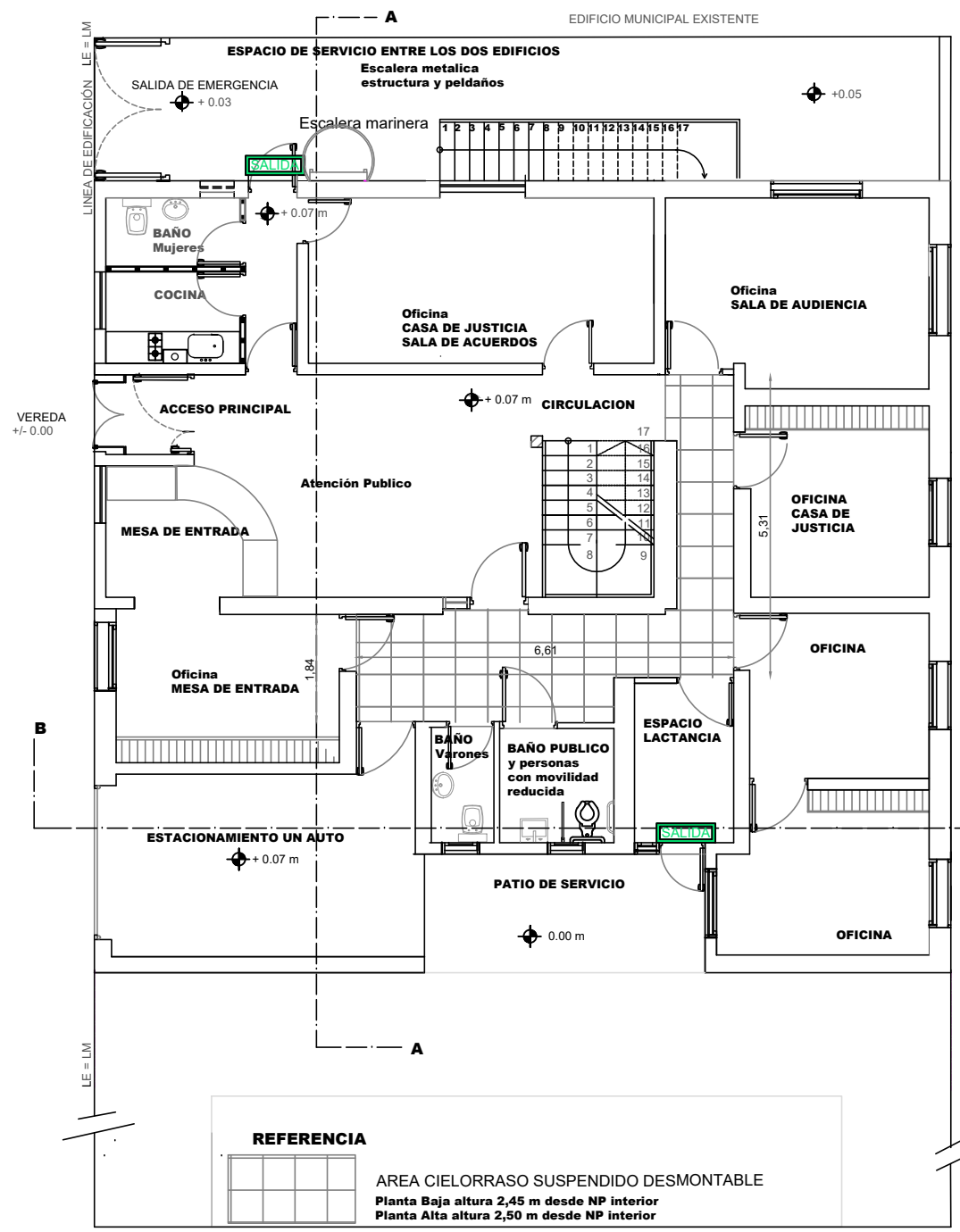
PLANTA BAJA
