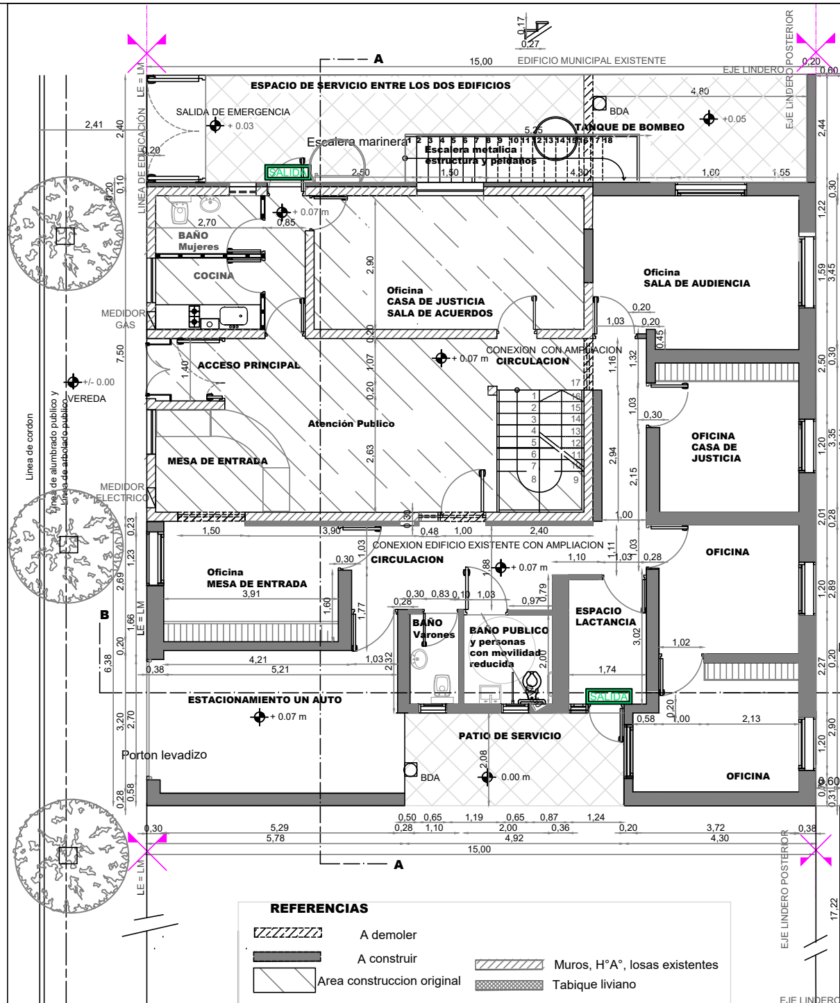
PLANTA BAJA
