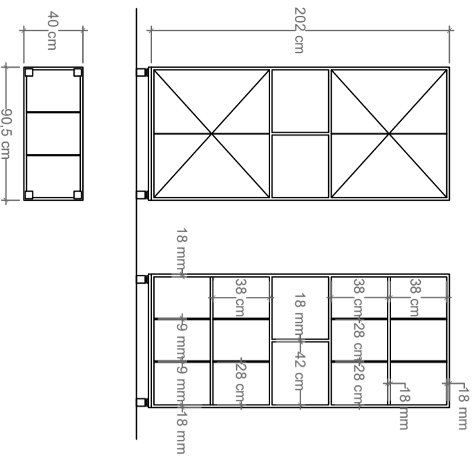
Ar-01 _ 7 unidades. Biblioteca alta con puertas de abrir.
