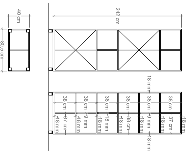
Ar-02 _ 2 unidades. Biblioteca alta con puertas de abrir.
