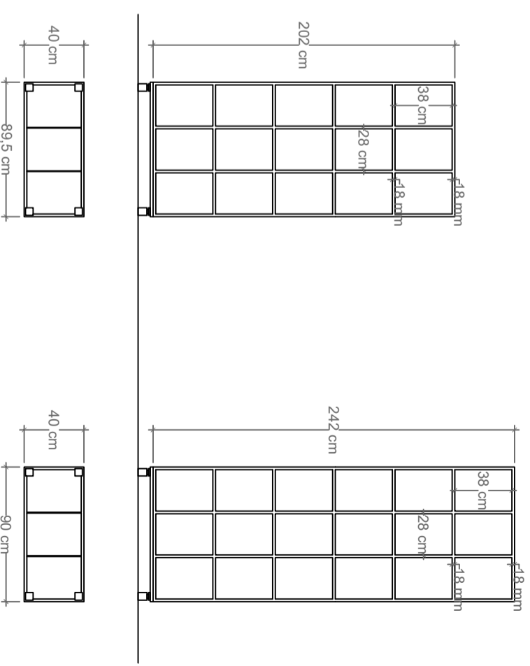
Ar-03 _ 4 unidades. Biblioteca alta con gabinetes.
