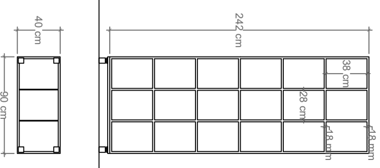
Ar-04 _ 4 unidades. Biblioteca alta con gabinetes.
