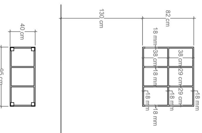
Ar-06 _ 1 unidad. Estantería flotante.
