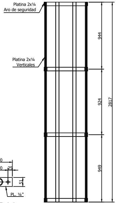
CORTE A-A
