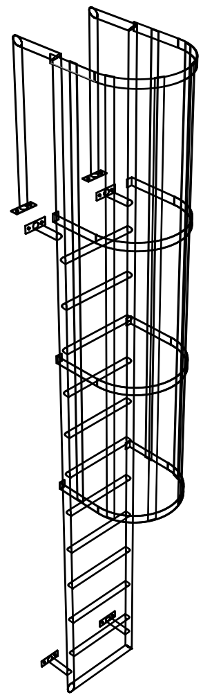
ISOMETRICO
