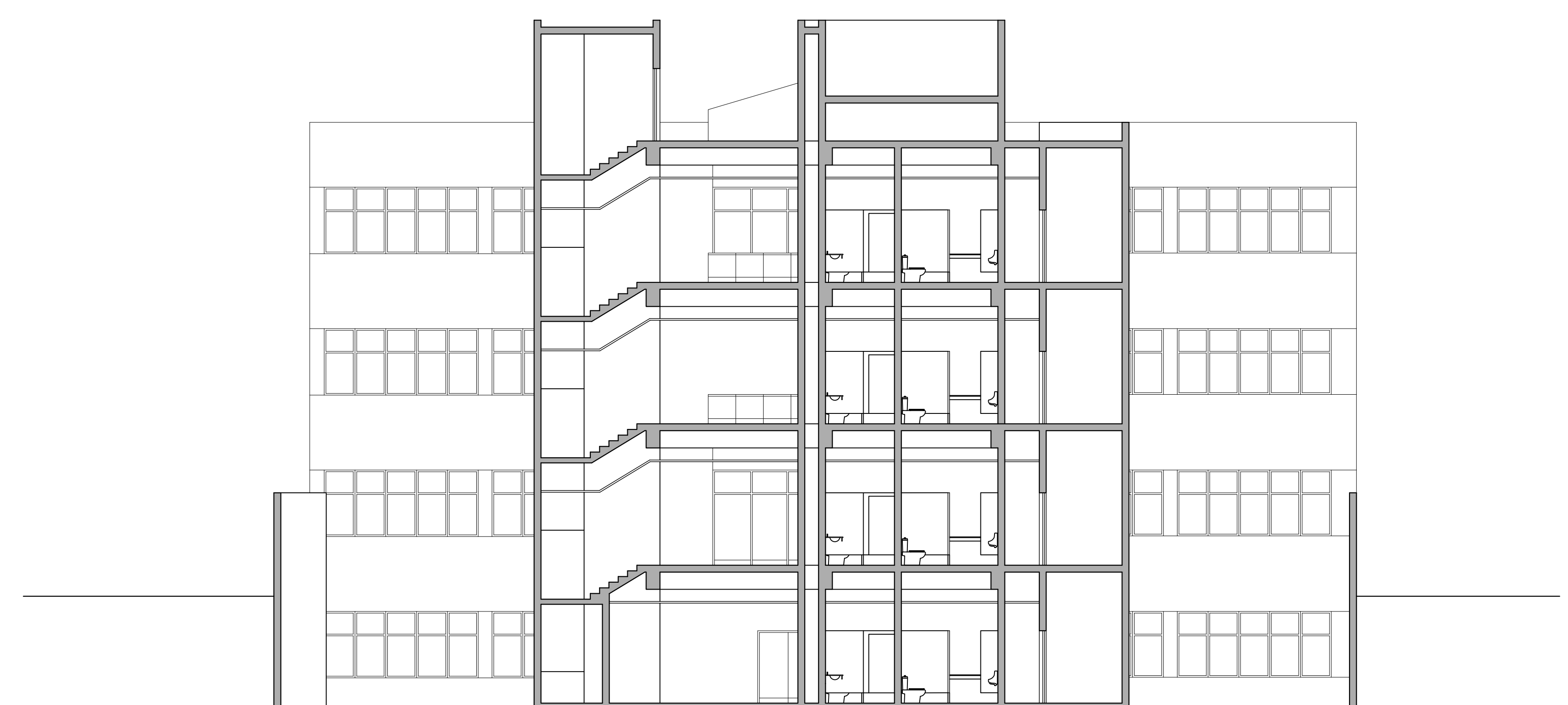
CORTE D-D
