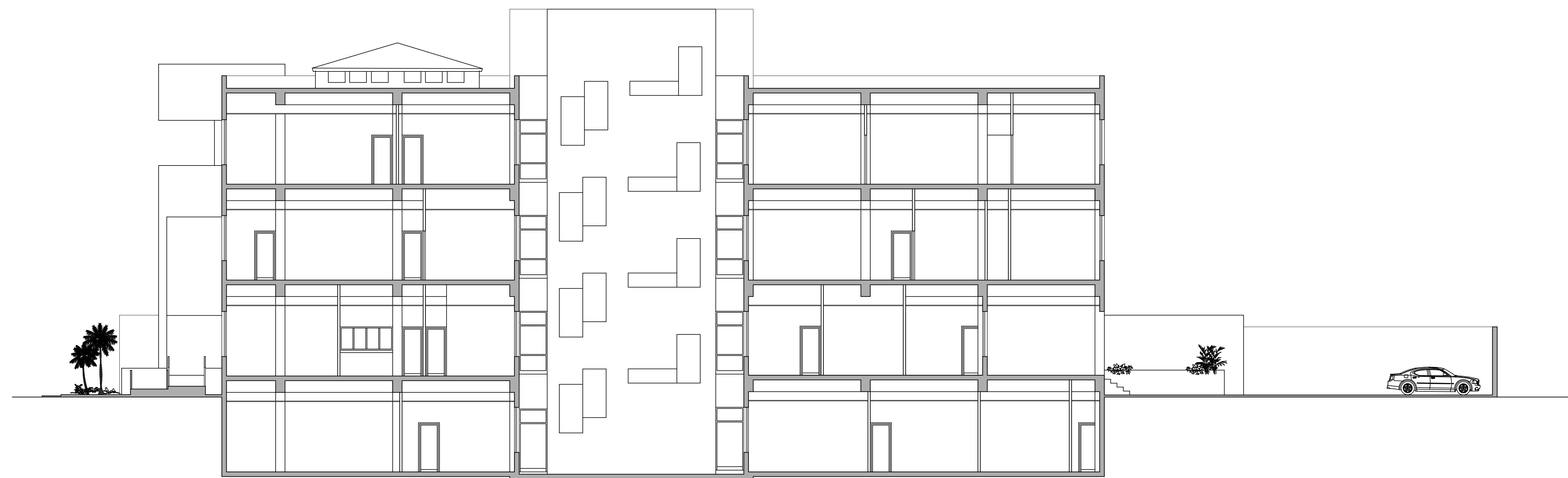
CORTE C-C
