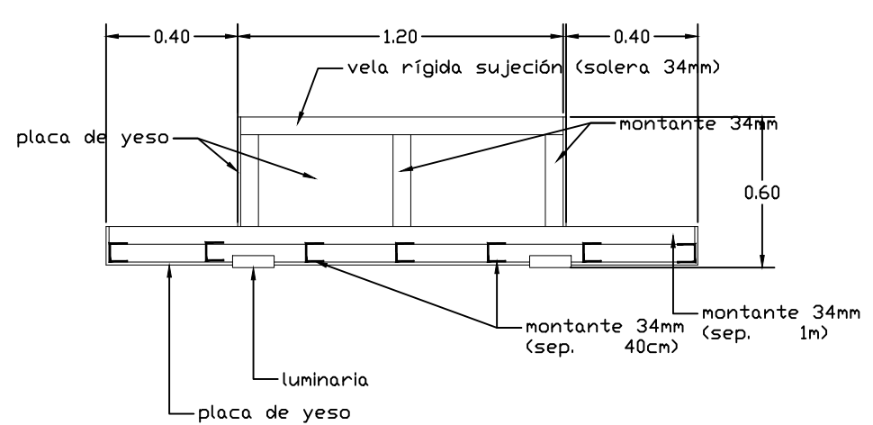
ESQUEMA ESTRUCTURA CIELORRASO SUSPENDIDO
