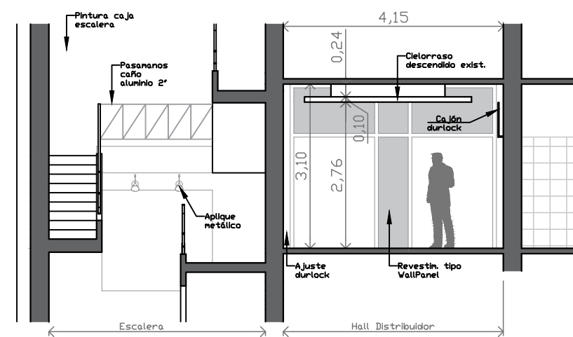
CORTE D-D
