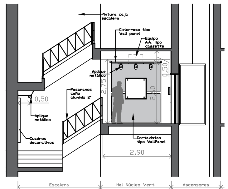
CORTE E-E
