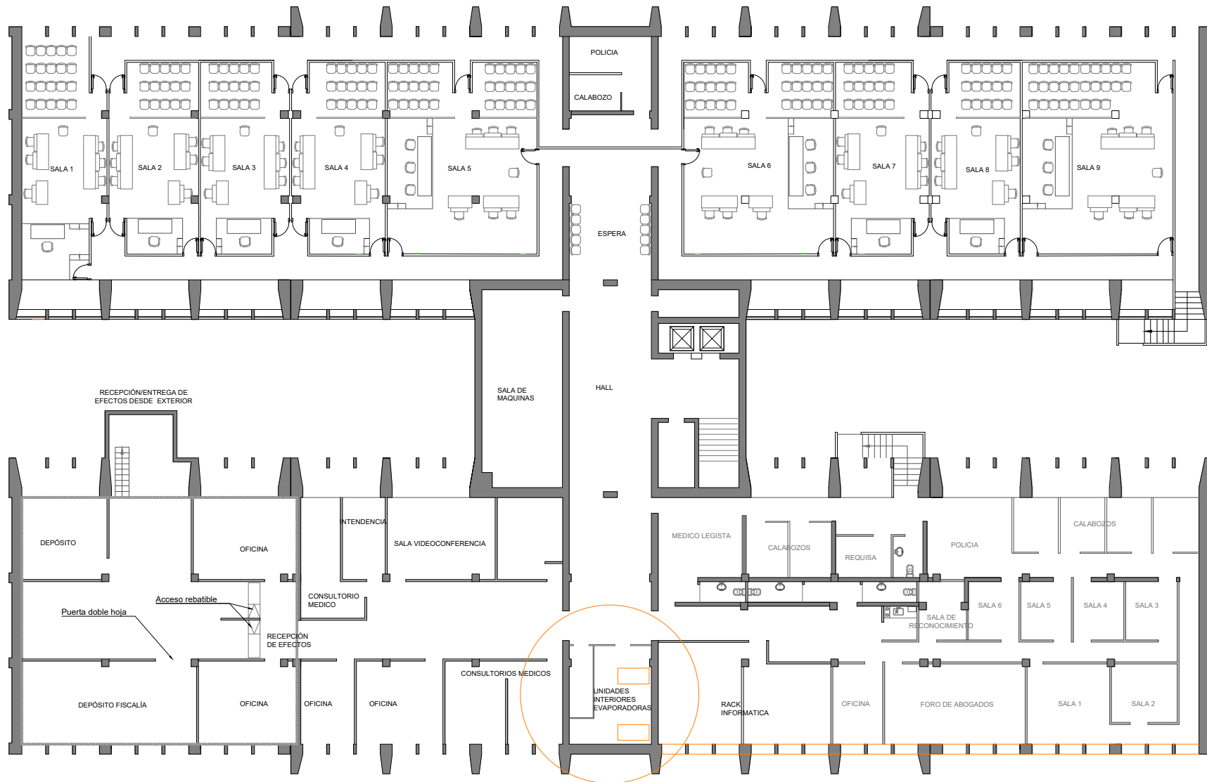
PLANTA SUBSUELO
