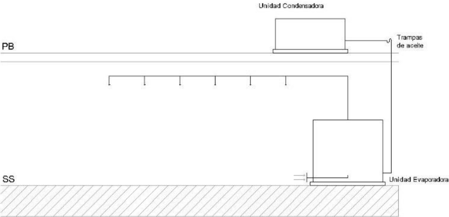
DISPOSICIÓN DE EQUIPOS DE FRÍO DE PRECISIÓN DATA CENTER PODER JUDICIAL DE SAN JUAN
