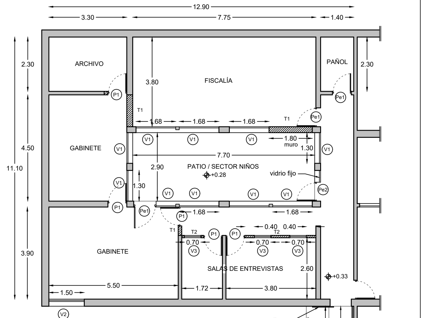
PLANTA SITUACIÓN PROYECTADA
