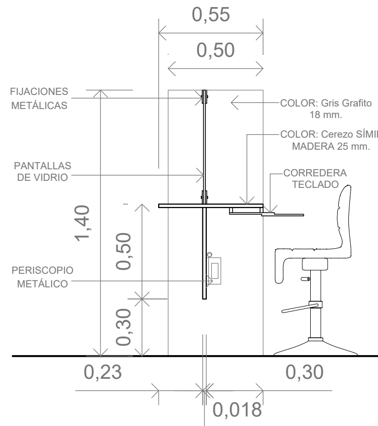
Corte Transversal
