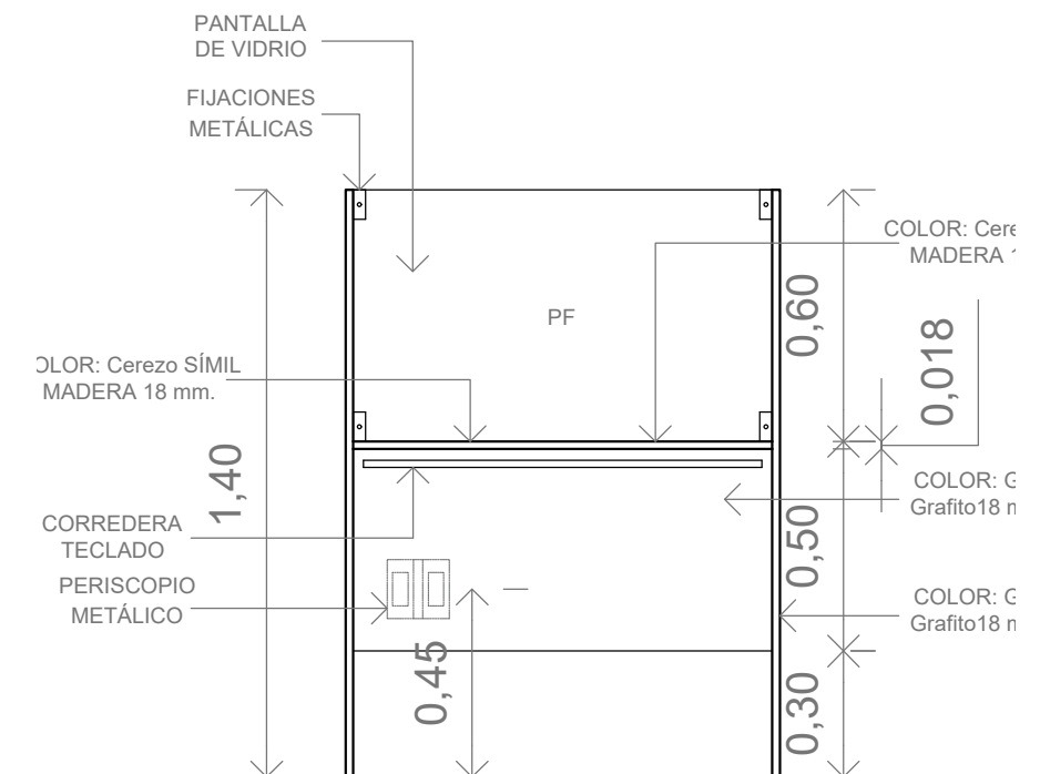
Vista Posterior
